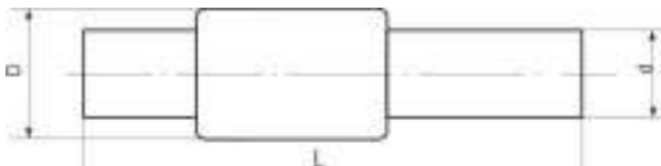
Рис. 2 Изолирующие соединения ИС-22...60
